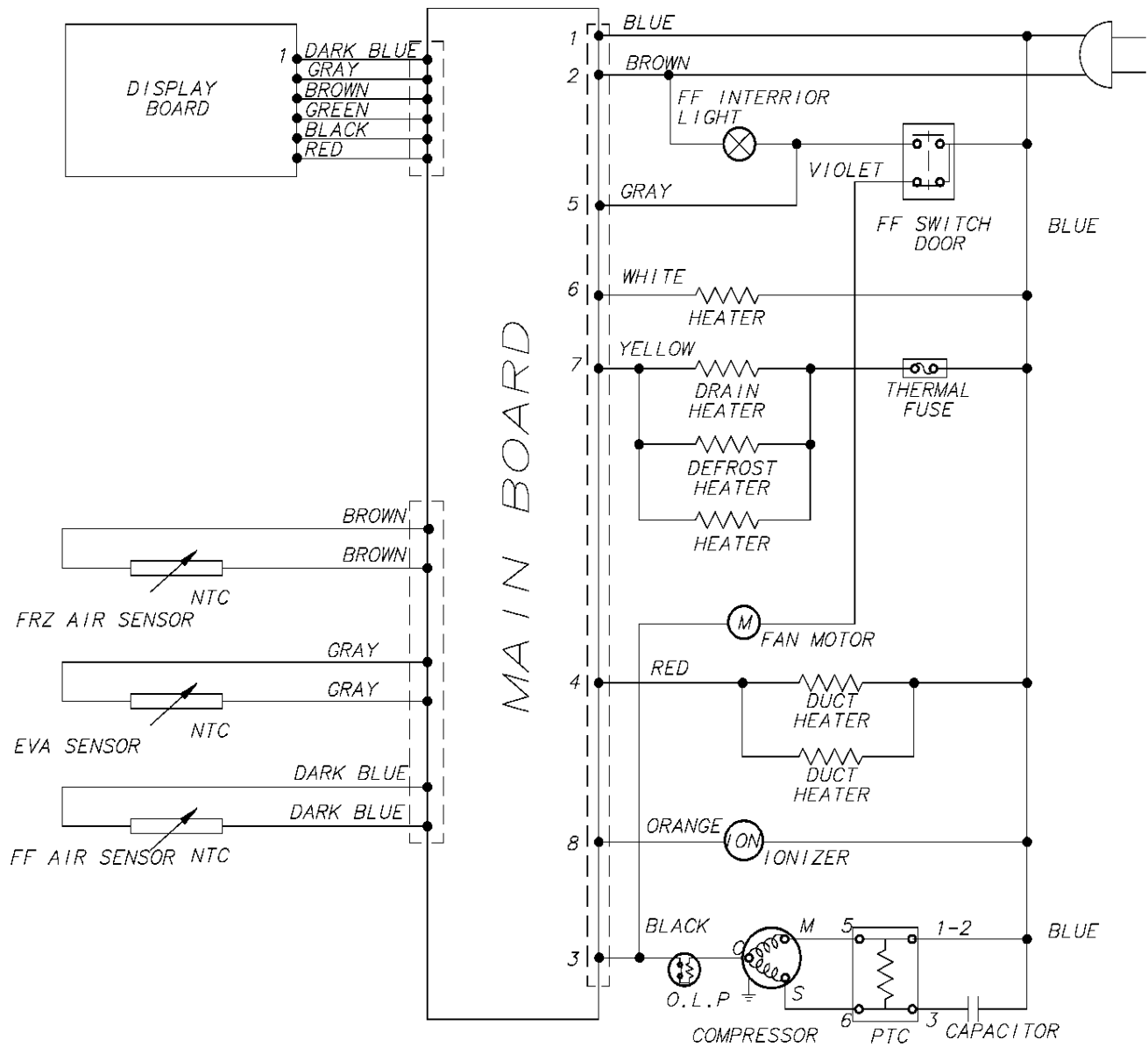
WIRING DIAGRAM (B-764)
