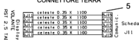
CONNETTORE: MODULO J11 / DISPLAY
