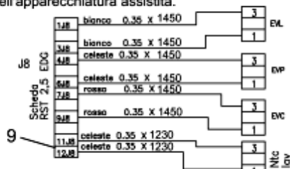
CONNETTORE: MODULO J8 / ELETTROVALVOLE (EVL - EVP-EVC) - Ntc
