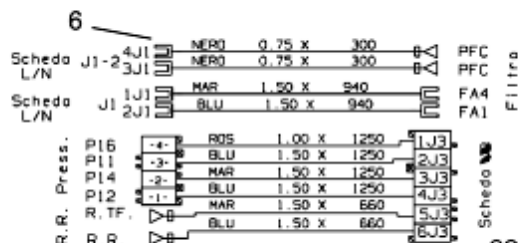
CONNETTORE: MODULO J3 / PRESSOSTATO - RESISTENZA MODULO J1-2 / FILTRO
