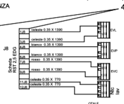
COD. C00143389 CONNETTORE: MODULO J8 / ELETTROVALVOLE (EVL - EVP-EVC) - Ntc
