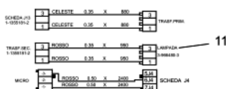
CONNETTORE: LUCE-TRASF-MICRIT. (MOD. J13 J4)
