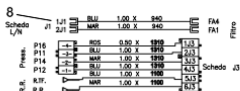
CONNETTORE: MODULO J3 / PRESSOSTATO - RESISTENZA MODULO J1/ FILTRO
