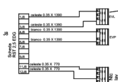
COD. C00143389 CONNETTORE: MODULO J8 / ELETTROVALVOLE (EVL - EVP-EVC) - Ntc
