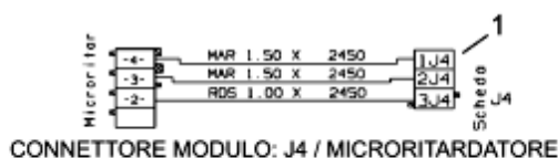
CONNETTORE MODULO: J4 / MICRORITARDATORE
