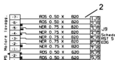
CONNETTORE MODULO J9 / MODULO POMPA DI SCARICO
