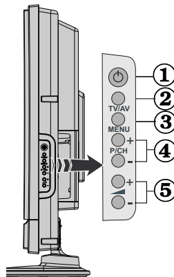
SEITENANSICHT
