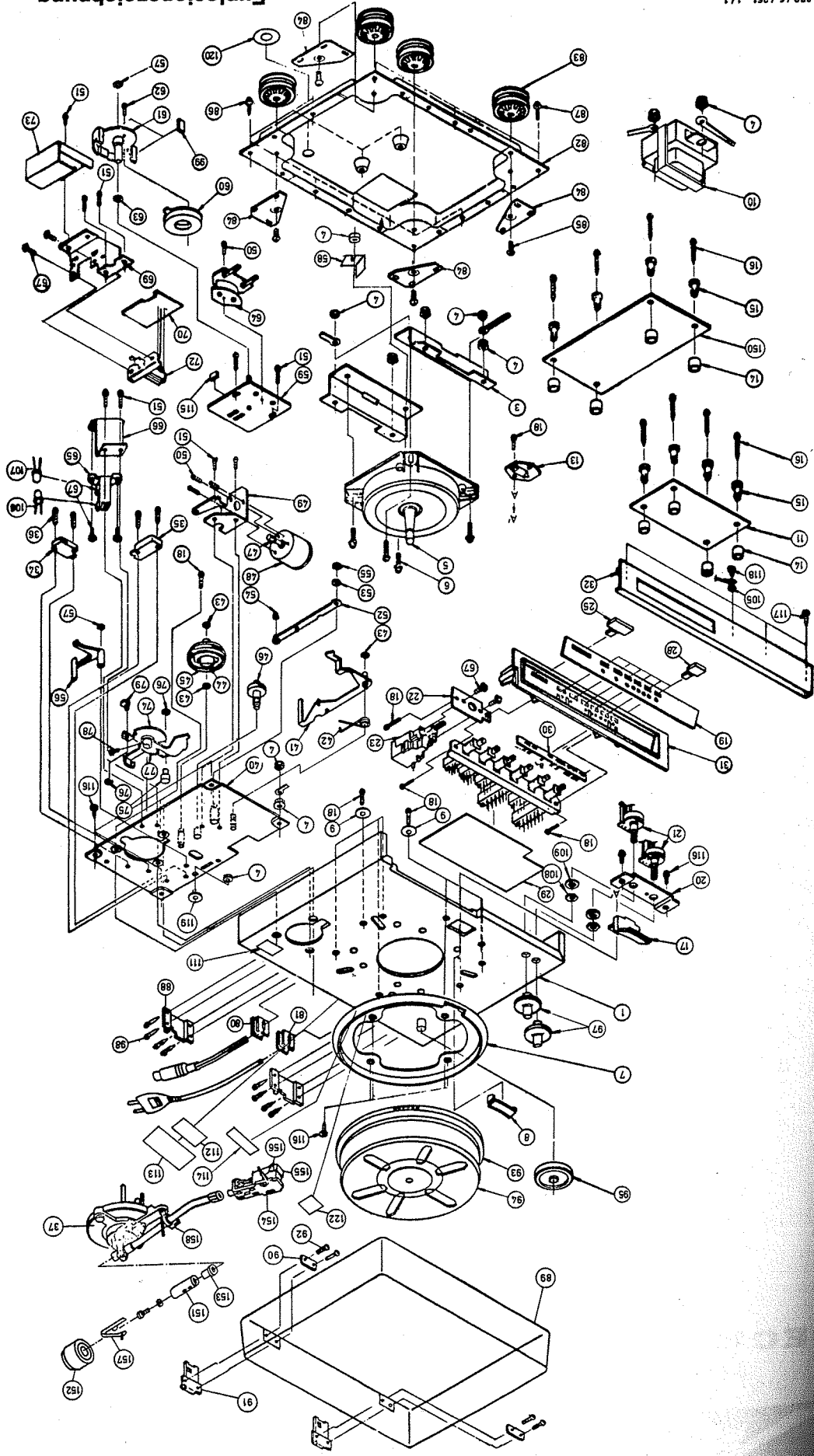
Explosionszeichnung Gerät TX 4963 kpl Exploded view Unit complete TX 4963
