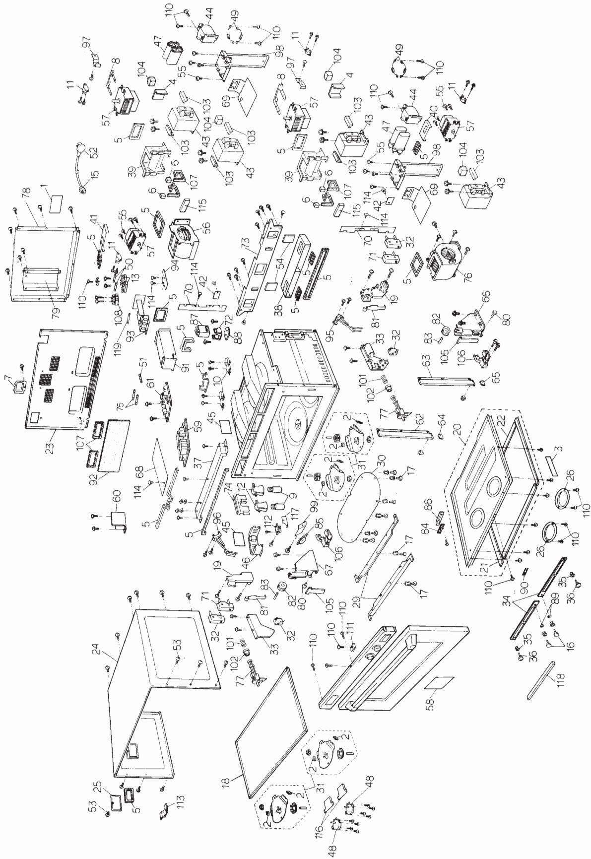
EXPLOSIONSZEICHUNG (EXPLODED VIEW)
