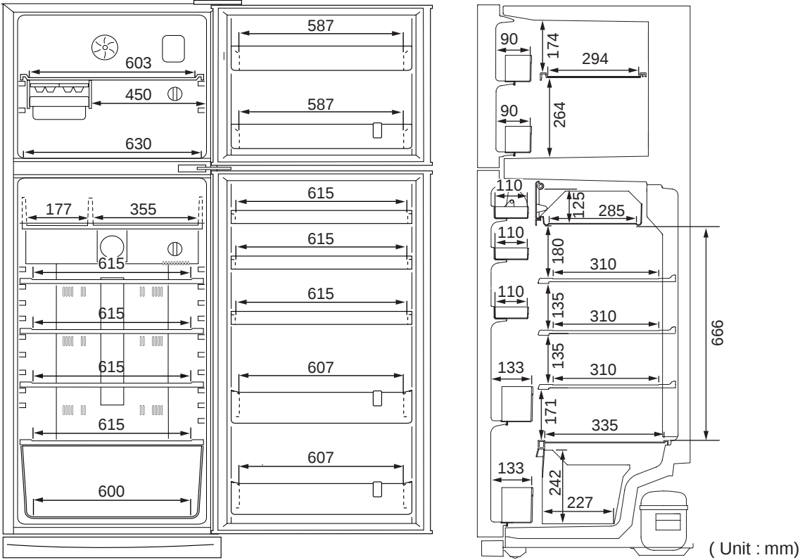
Fig. E-2 (SJ-PK60M,K60M,PK65M,K65M)
