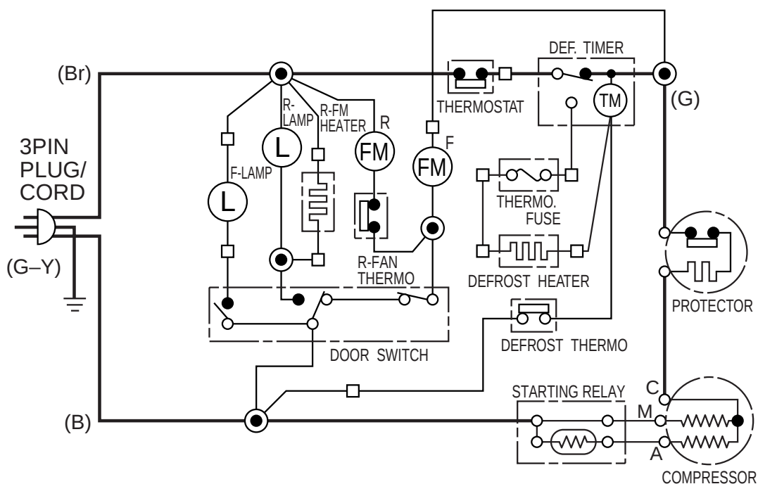
Figure W-2. Wiring Diagram (SJ-K60M,K65M,K70M)
