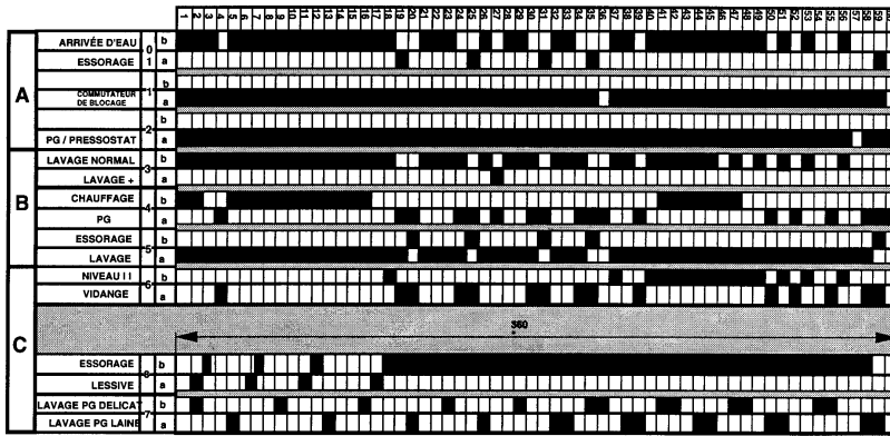
DIAGRAMME ML 4600 (commun à plusieurs type de lave linge) Pour PG : Type : EC 4439 - EATON
