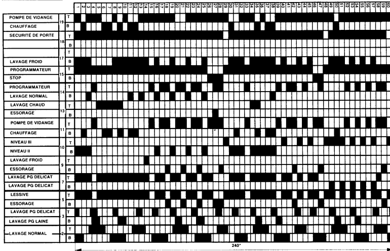
DIAGRAMME ML 4600 (commun à plusieurs type de lave linge) Pour PG : Type T 2000 - CROUZET
