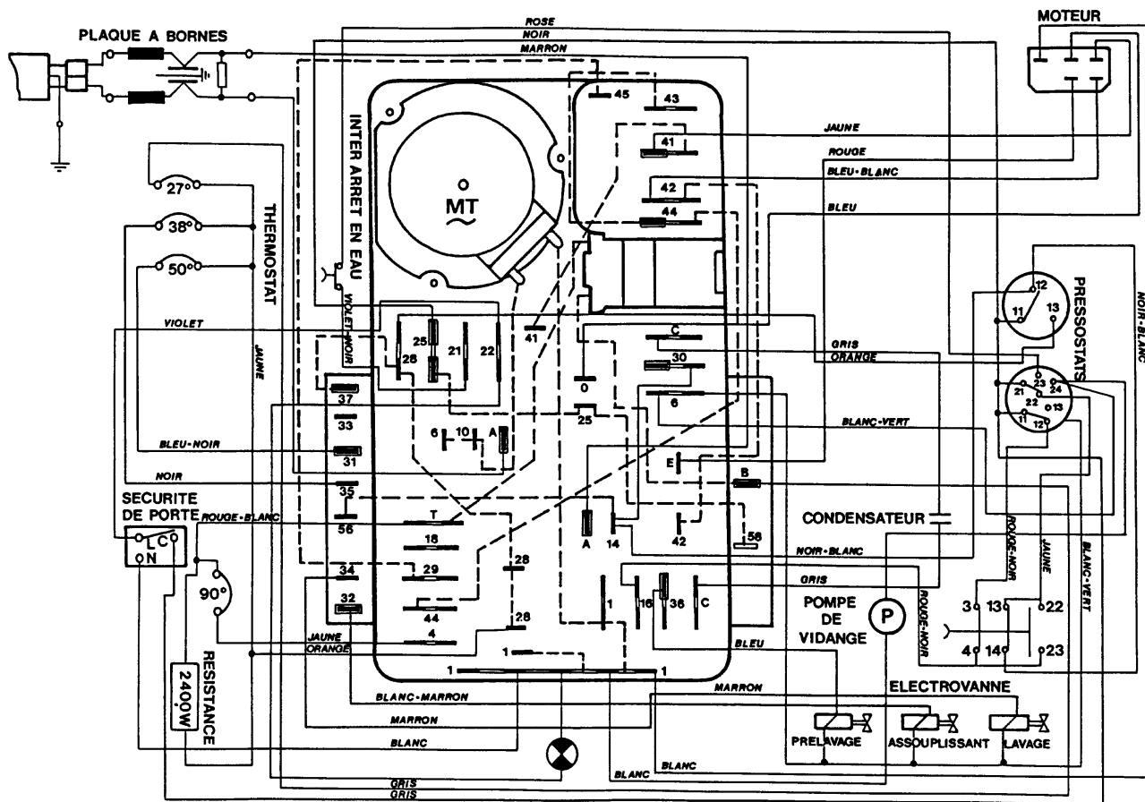
SCHEMA DE CABLAGE PROGRAMMATEUR EATON 9095
